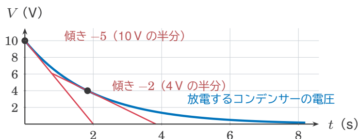
図8 例題3の放電のグラフ（式は6-4で求める）。どの点でも、接線の傾きは「今の電圧の半分」で下向き。
