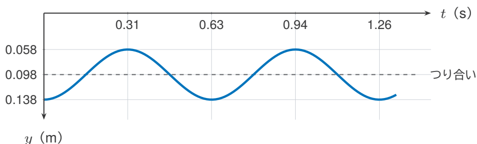
図5 つり合いの位置から 4 \text{ cm} 引いてはなしたおもりの位置 y （下が+なので、グラフの下向きを+にした）。ゆれの中心は y_0 = 0.098 \text{ m} 。
