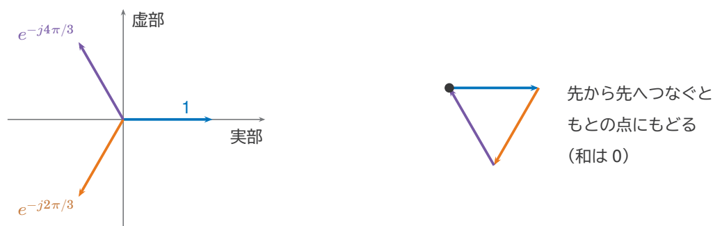
図7 三相交流のフェーザ。左：120° ずつずれた3本の矢印。右：つなぐと正三角形になり、和は0。
