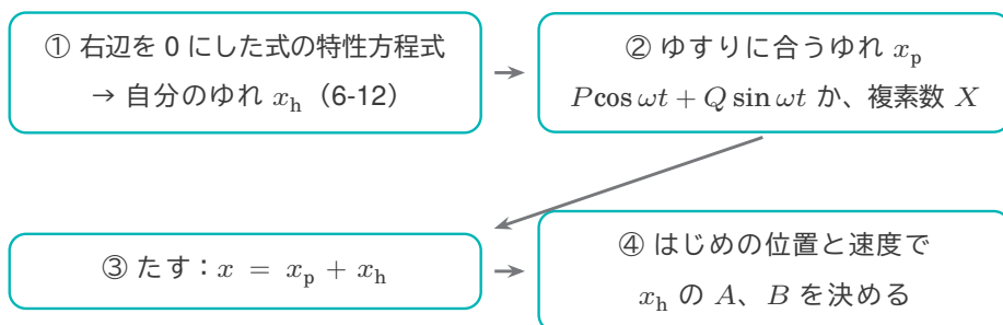
図7 ゆすられる式は、この順で解く。共振のようすだけ知りたいときは、②の |X| だけを見ればよい (自分のゆれは、やがて消えるから)。
