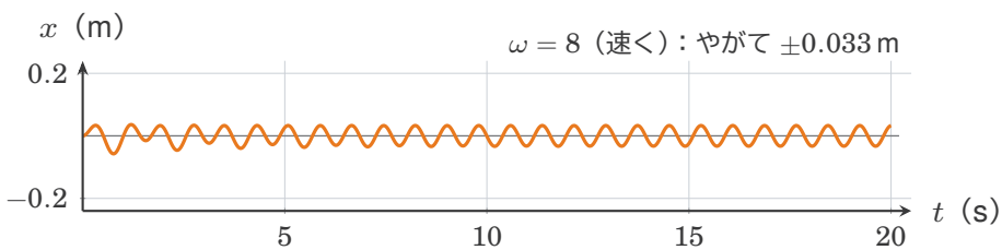
図4 速く ( \omega = 8 ) ゆすった。たての目もりは、図3の \omega = 2 のグラフと同じ。
