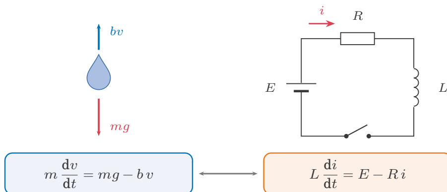
図7 左：速さに比例する抵抗を受けて落ちる物。右：RL 回路。2つの式は、文字を入れかえると同じ形になる。
