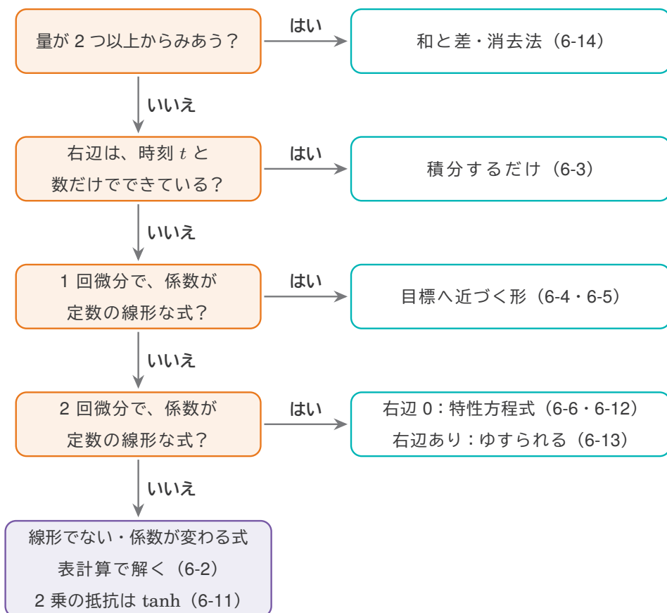
図5 解き方の地図。どの道に進んでも、表計算(6-2)なら必ず数で解ける。式で解いたら、表計算の結果と重ねて確かめる。
