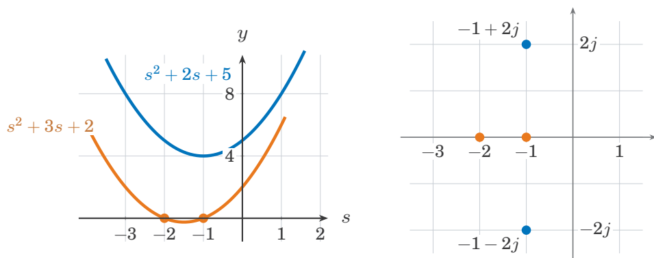
図4 左: y = s^2 + 3s + 2 (オレンジ) は横軸と -2 、 -1 で交わる。 y = s^2 + 2s + 5 (青) は交わらない。右: 解を平面にかく。 D > 0 の解 (オレンジ) は横の線の上、 D < 0 の解 (青) は線の外に、上下対称にある。
