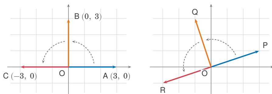
図1 左：Aを90°ずつ2回回すと、Cは-3。右：Pを2回回したRは、Pと原点について反対の位置。
