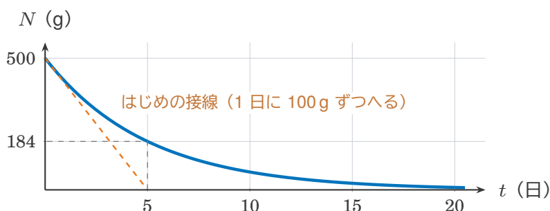
図 11 N = 500e^{-0.2t} 。はじめの速さ (1日に 0.2 \times 500 = 100 g) のままなら 5 日 ( \tau ) で 0。じっさいは 5 日で 37% (184 g) 残る。
