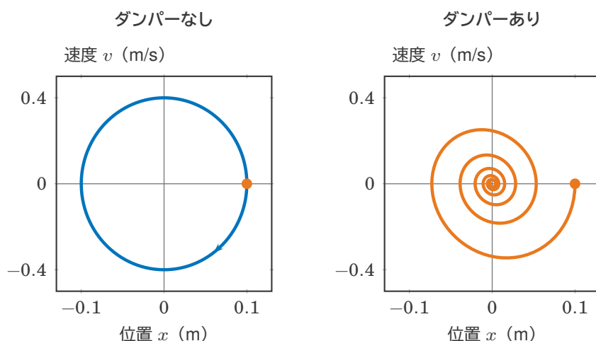
図7 状態の点 (x, v) の動き (6-6・6-7 のばね: 0.5 kg、8 N/m、はじめ x = 0.1 m、 v = 0 。オレンジの点がスタート)。ダンパーなし: 同じだ円を回り続ける。ダンパーあり ( c = 0.4 N・s/m): うずをまいて原点 (止まった状態) へ近づく。
