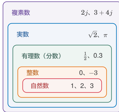
図3 左：複素数は平面の点。横の線の上が実数。右：数の仲間。外側の箱ほど広い。
