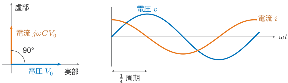
図 8 コンデンサーの電圧と電流。左：フェーズ。電流の矢印は、電圧の矢印より 90^\circ 先にある。右：電流の山（オレンジ）は、電圧の山（青）より \frac{1}{4} 周期早く来る。
