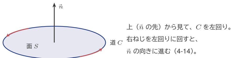
図9 道 C を回る向きと、面 S の向き \vec{n} は、右ねじの関係にとる。
