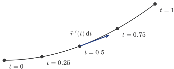
図4 道の上の場所に、時刻 t の目もりをつける。時刻 t の所から短い時間 dt に動く矢印は、速度 \vec{r}'(t) に dt をかけたもの。
