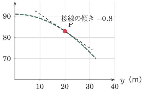
図 3 2 つの切り口のグラフ。黒い点線は P での接線。東西の切り口の傾きは -0.6 、南北の切り口の傾きは -0.8 (⑥で計算する)。
