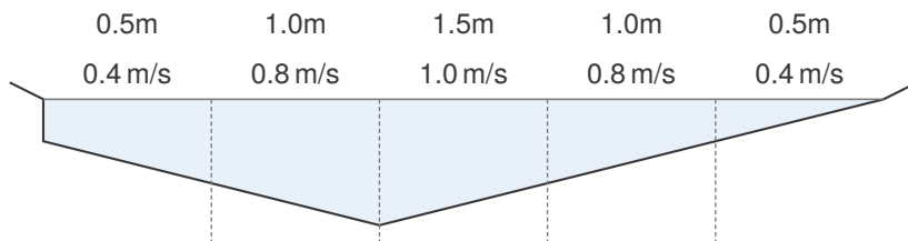
図 14 川の断面 (深さは見やすいように大きくかいた)。区間ごとに、深さと平均の速さを測る。
