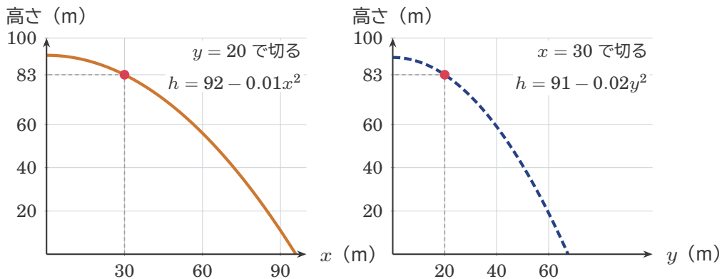
図8 2つの切り口。左は北へ20 mの所を東西に、右は東へ30 mの所を南北に切ったもの。どちらも、点(30, 20)の上の83 m(赤い点)を通る。
