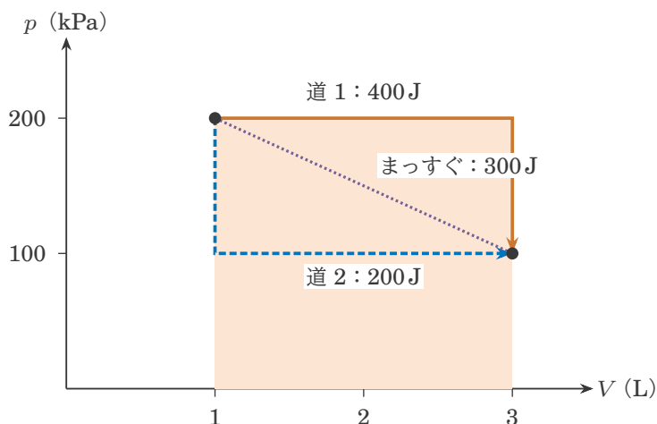
図 6 p - V 図の上の 3 つの道。どれも 1 \text{ L} \cdot 200 \text{ kPa} の状態から 3 \text{ L} \cdot 100 \text{ kPa} の状態へ。気体がする仕事 \int p dV は、道の下面積で、道によって変わる（例題 11）。
