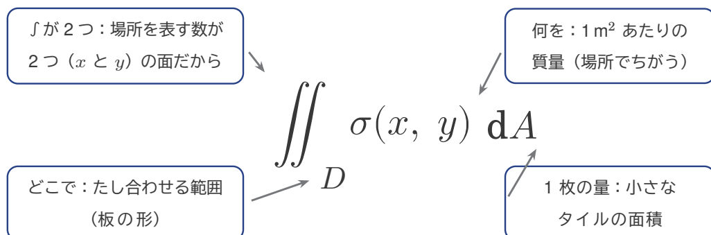
図3 重積分の記号の読み方。
