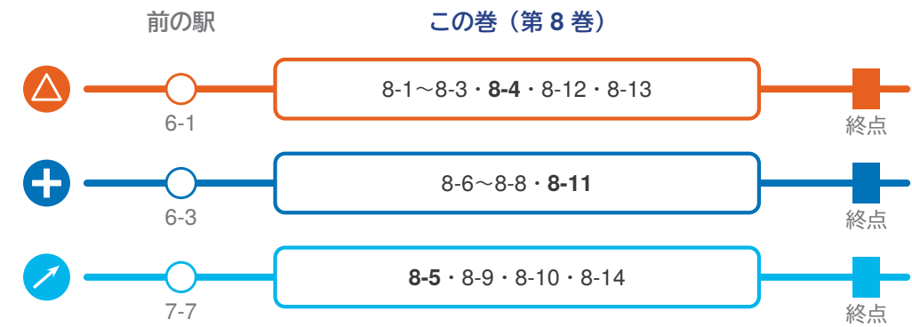
図 10 第 8 巻を通る 3 本の路線。四角の中がこの巻の駅（太字が終点の駅）。右はしの四角が終点の印。終点は、その路線の大きな目的地。終点のあとの駅（8-12 など）は、終点で作った道具を使う駅。
