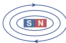
(2) 磁力線は、いつも輪になる
