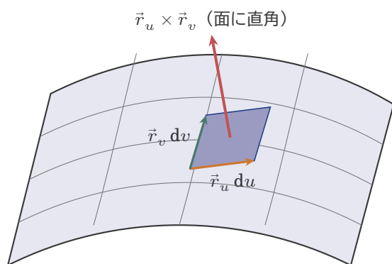
図8 曲がった面を、 u の線と v の線で区切ると、小さな平行四辺形のタイルができる。2本の辺の矢印の外積が、タイルの向きと面積を一度に表す。
