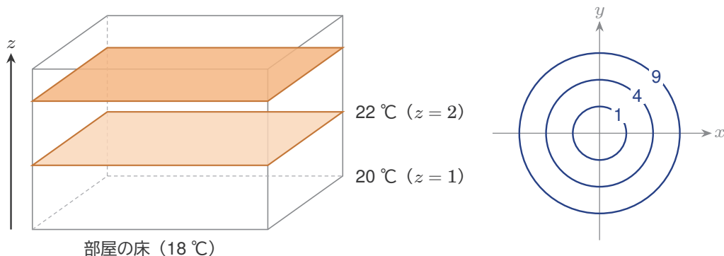
図9 左: T = 18 + 2z の部屋の、 20\text{°C} と 22\text{°C} の等値面 (水平な面)。右:
