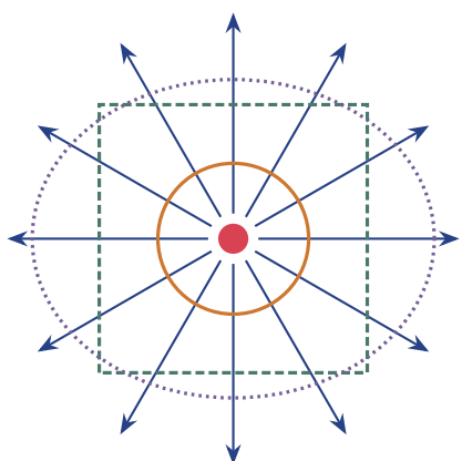
図12 点電荷を囲む、形のちがう3つの袋（切り口）。袋の形を変えても、電荷から出る線はすべて袋を通りぬける。
