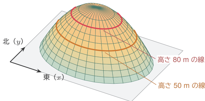
図 2 主役の山の鳥瞰図（南東の空から見下ろした図）。山の面の横の輪が、10 m ごとの「同じ高さの線」。赤は 80 m、オレンジは 50 m。
