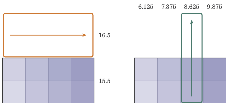
図4 行の合計（オレンジのわく）は、 y を1つに止めて、横にならんだタイルをたしたもの。列の合計（緑のわく）は、 x を止めて、たてにたしたもの。
