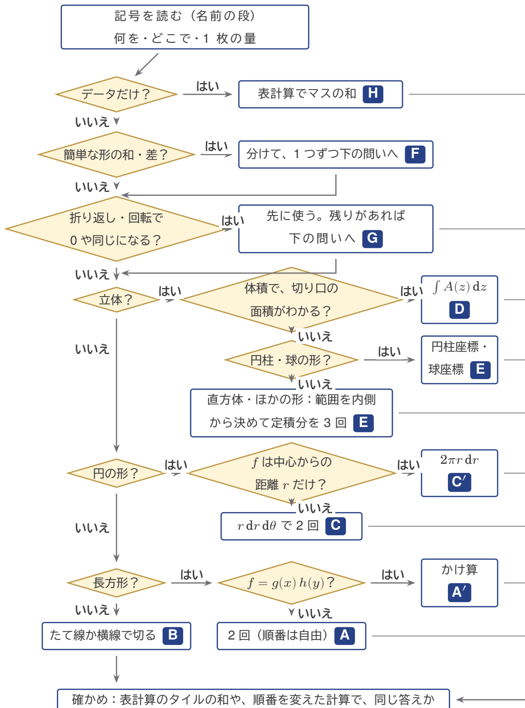
図5 重積分の流れ図。ひし形は問い、四角はすること。上の3つの問い（H・F・G）が楽をする段、下が直す段。F・Gのあとは左の列の次の問いへもどる（Gで答えが全部決まったときは、右の線へ）。計算した四角からは、右の線をたどって最後の「確かめ」へ。
