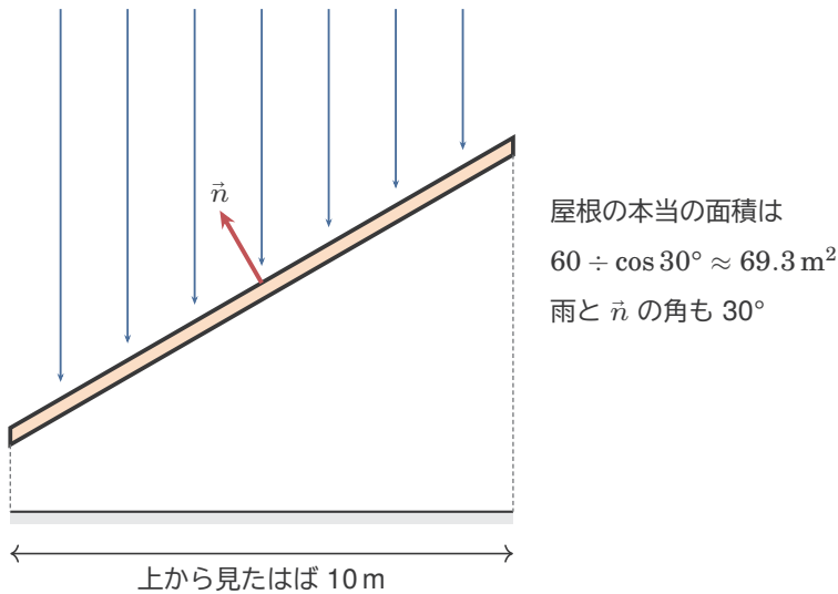
図4 30° かたむいた屋根（横から見た図）。屋根の本当の面積は大きいが、雨は面にななめに当たる。
