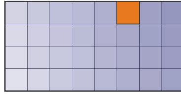
8-6：面のタイル（面積 dA ）
