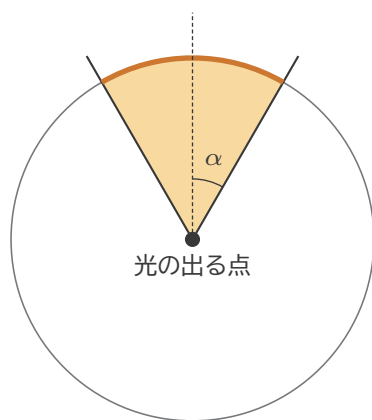
図13 円すいの立体角。光の出る点を中心とする半径1の球面のうち、円すいの中にある「おわん」の部分の面積が、立体角。
