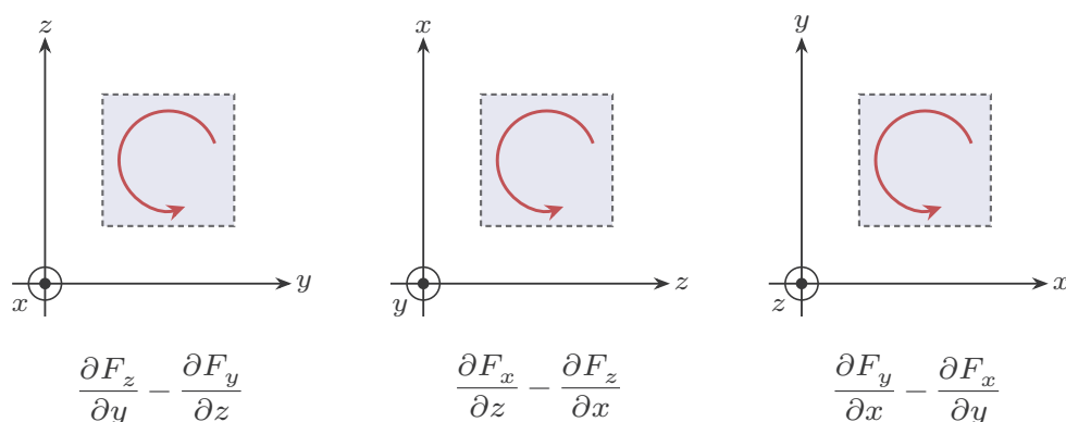
図7 左から、 x 軸・ y 軸・ z 軸のまわりの回り方。どの図も、残りの軸（原点の \odot ）が紙の手前に向かっていて、手前から見て左回りが正（右ねじが進む向き：4-14）。
