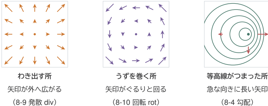
図 4 矢印の地図から読みとれる 3 つのこと。右の図は、頂上（緑の点）が右によった山の等高線。赤い矢印はボールの転がる向き（勾配 grad の反対の向き）で、線の間がせまいほど坂が急で、矢印が長い。
