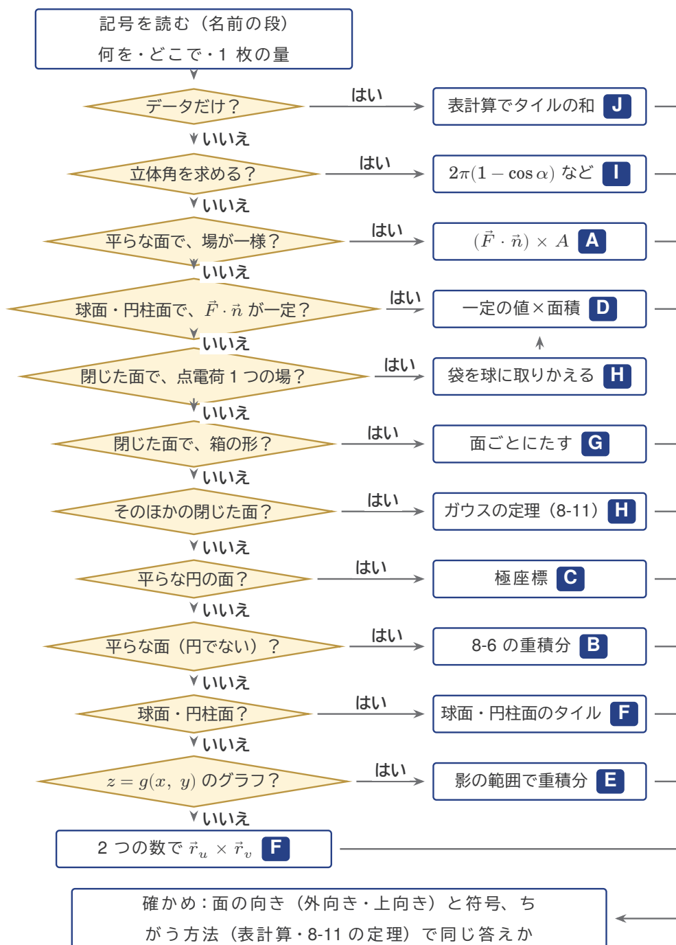
図7 面積分の流れ図。ひし形は問い、四角はすること。上の問い (J・I・A・D・H・G) で楽な道をさがし、下の問い (C・B・F・E) で面の形から直し方を選ぶ。向きのいない量では「 f が一定?」と読む。「点電荷1つの場」は、わき出しが1点の電荷だけの場 (電荷が中なら球に取りかえて D、外なら 0)。どの四角からも、右はしの線を通して「確かめ」へ。
