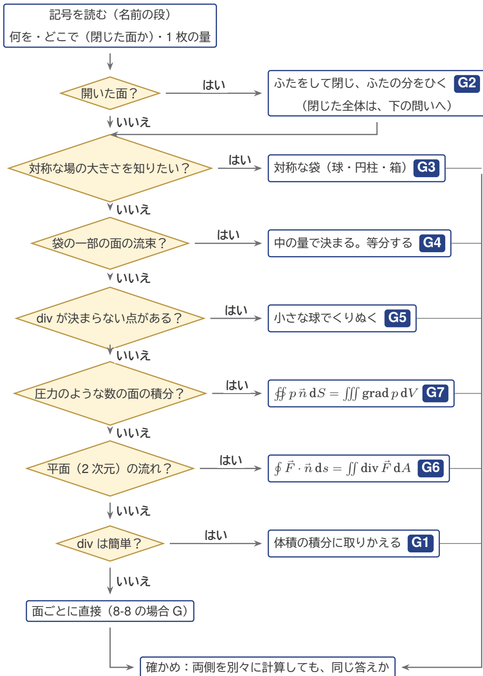
図5 ガウスの定理を使うときの流れ図。ひし形は問い、四角はすること。上から順に答えて、はいなら右の四角へ。どの四角からも、最後は「確かめ」へ進む。
