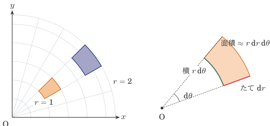
図7 左：極座標のタイル。同じ dr \cdot d\theta でも、中心から遠いタイル(紺)は、近いタイル(オレンジ)より大きい。右：タイル1枚を大きくした図。たては dr 、横は半径 r の円の弧で r \, d\theta 。
