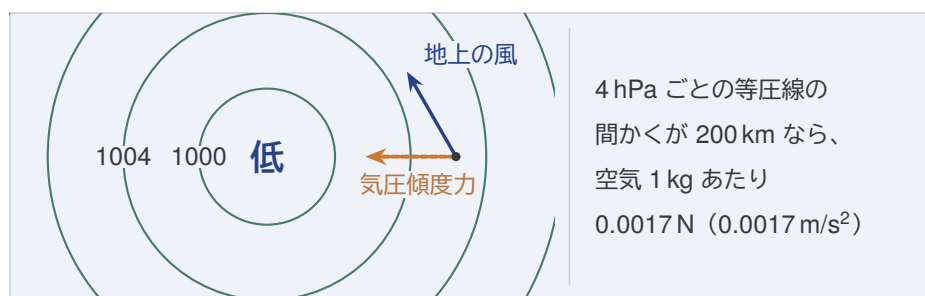
図8 北半球の低気圧のまわり（模式図）。気圧傾度力（オレンジの点線）は等圧線（緑の線）と直角に低気圧へ向くが、地上の風（紺の矢印）は右へそれ、等圧線をななめに横切って吹きこむ。
