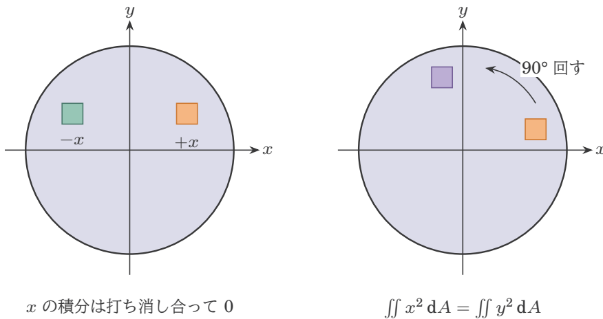
図 10 円の板の対称性。左： y 軸で折り返すと x の符号が変わるので、 x をたすと 0。右： 90^\circ 回すと x と y が入れかわるので、 x^2 をたしても y^2 をたしても同じ。
