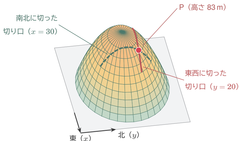
図2 主役の山を東の空から見た図に、P を通る2枚の板で切った切り口をかいだ。赤の線は東西の板 ( y = 20 ) の切り口、緑の点線は南北の板 ( x = 30 ) の切り口 (赤の線は、山の向こう側にかくれる所をかいていない)。
