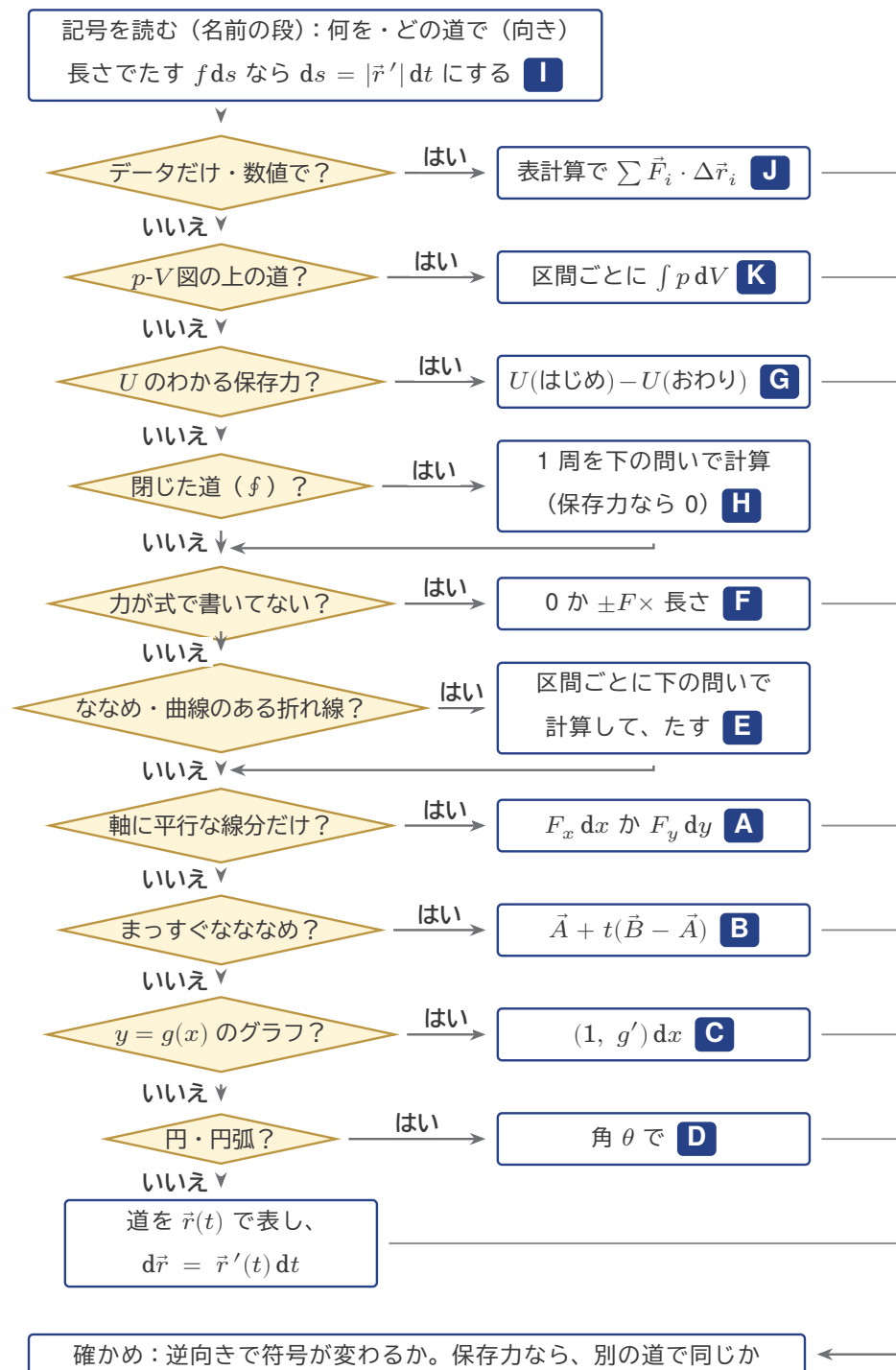
図 3 線積分の流れ図。ひし形は問い、四角はすること。上の 5 つの問い（J・K・G・H・F）が楽をする段、下が直す段。H・E のあとは左の列の次の問いへもどる。計算した四角からは、右の線をたどって最後の「確かめ」へ。
