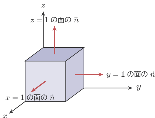
図 11 立方体の箱。見えている3つの面 ( x=1 \cdot y=1 \cdot z=1 ) の外向きの \vec{n} は、それぞれ x \cdot y \cdot z の正の向き。見えない3つの面 ( x=0 \cdot y=0 \cdot z=0 ) の \vec{n} は、負の向き。
