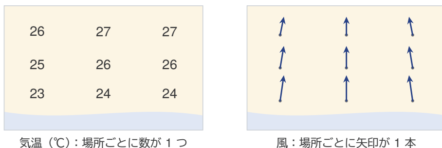
図1 同じ町の、夏の昼の気温の地図と風の地図 (模式図。下の青い所は海で、海から陸へ海風がふく)。風の矢印の根もとの点が、その風をはかった場所。
