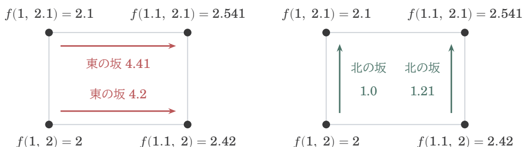
図6 f = x^2y の、4つの角の値。左：下の辺と上の辺で東の坂を求めた。右：左の辺と右の辺で北の坂を求めた（どちらも差を0.1でわった）。
