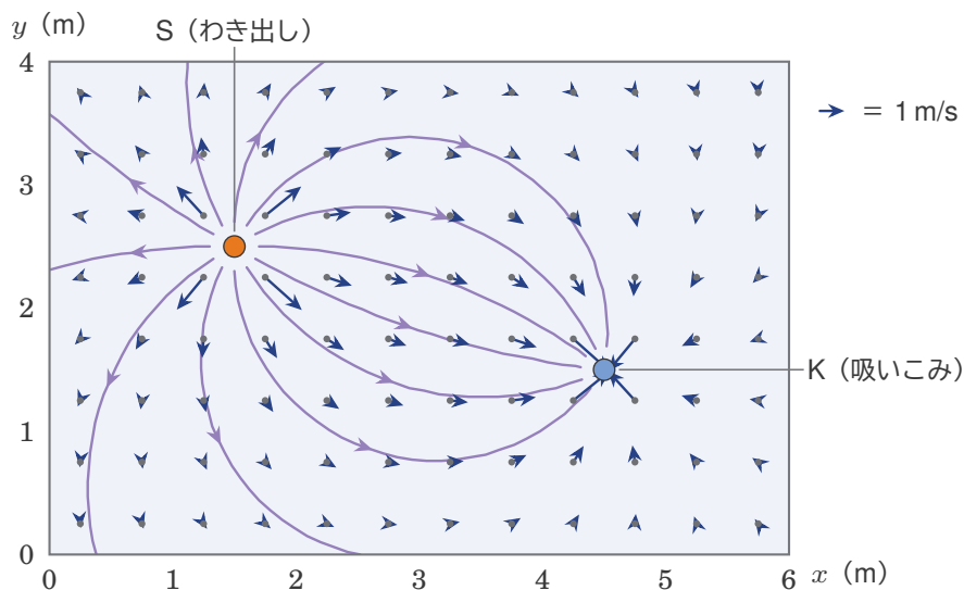
図4 池の流れ（矢印の根もととの点、その場所。0.5 m ごと）。むらさきの線は流線で、S から出て K に入る。
