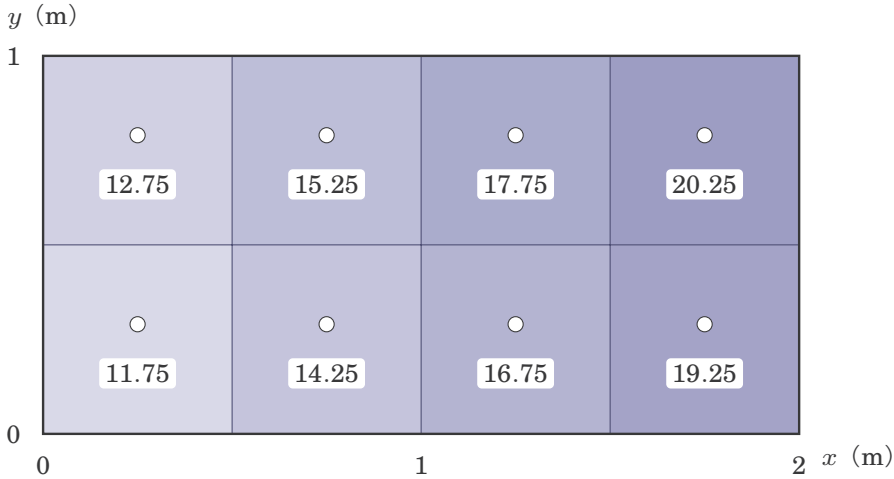
図1 8枚のタイルと、まん中の点（白い丸）の \sigma ( \text{kg/m}^2 )。たとえば右上のタイルは、 x = 1.75 、 y = 0.75 で \sigma = 10 + 5 \times 1.75 + 2 \times 0.75 = 20.25 、質量は 20.25 \times 0.25 \approx 5.06 \text{ kg} 。
