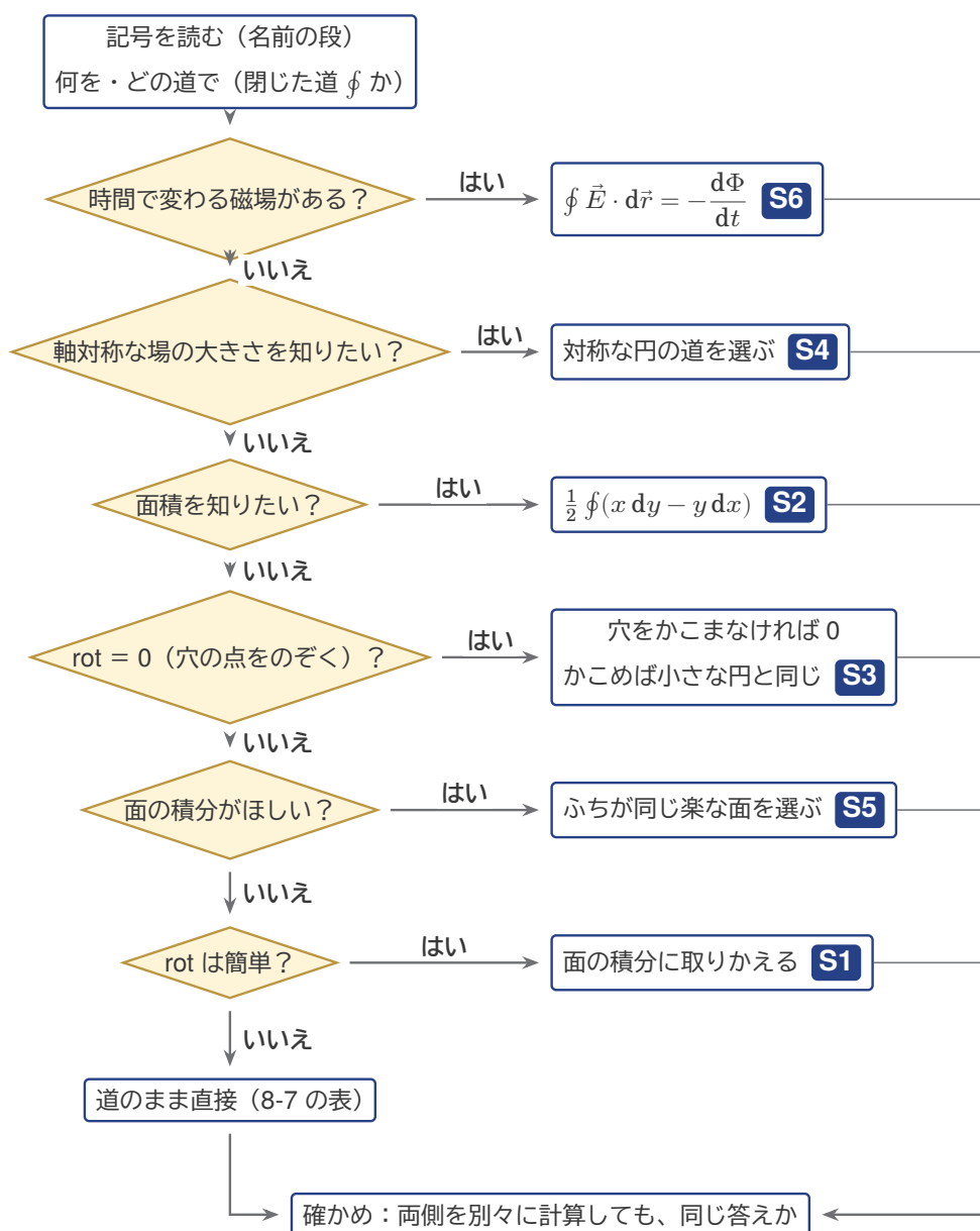
図 10 ストークスの定理を使うときの流れ図。ひし形は問い、四角はすること。どの四角から、最後は「確かめ」へ進む。時間で変わる磁場 (S6) の意味は 8-14 で読む。
