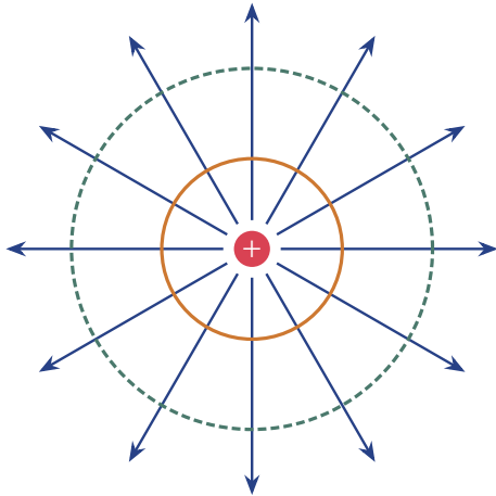
図 10 点電荷のまわりの電気力線（12 本だけかいた）。どの球も、同じ本数の線を受ける。 流束が半径によらないのは、このため。
