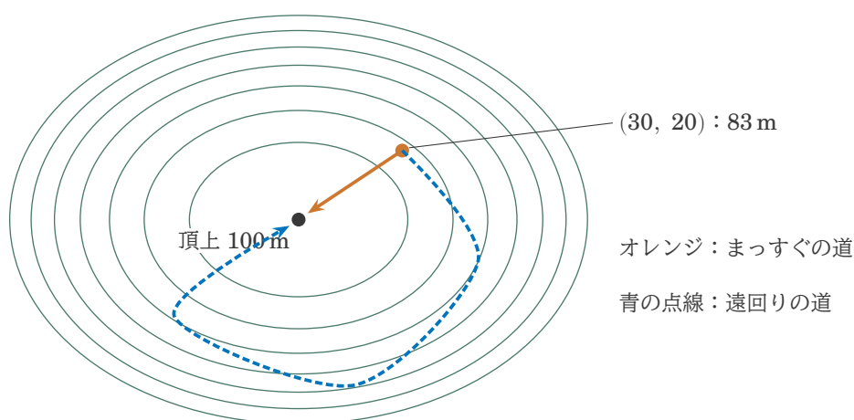
図5 主役の山を登る2つの道。重力は保存力なので、どちらの道でも、重力に逆らってする仕事は mg \times (100 - 83) で同じ。遠回りすると、坂がゆるやかになって必要な力は小さくなるが、進む距離が長くなる。
