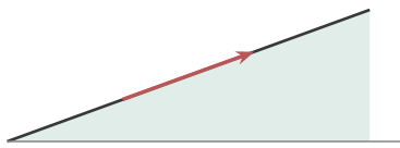
道が 1 本：坂の急さは 1 つの数 (傾き = 上がった高さ ÷ 進んだ長さ)
