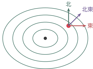
山の斜面：向きで坂の急さがちがう
