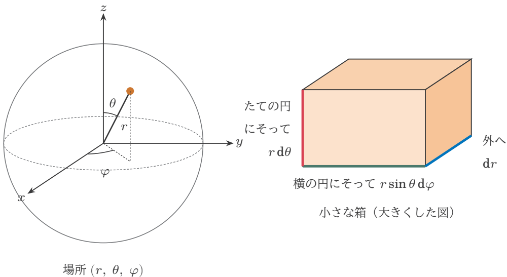
図 9 球座標の小さな箱。3 つの辺の長さをかけると、体積 dV = r^2 \sin \theta dr d\theta d\varphi 。
