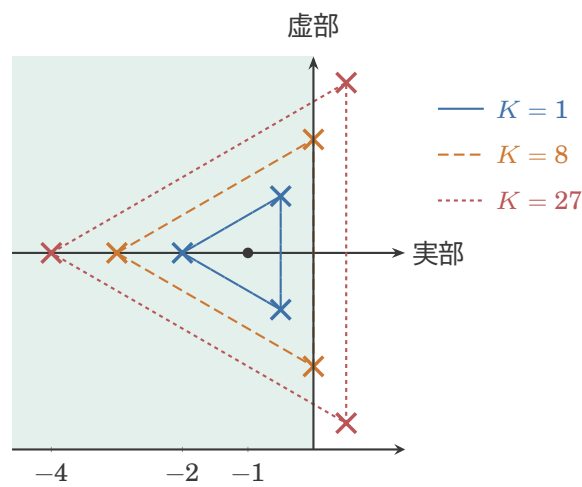
図 12 (s + 1)^3 + K = 0 の極 ( K = 1 は青の実線、 K = 8 はオレンジの破線、 K = 27 は赤の点線の三角形。うすい緑は左半分)。 K を大きくすると、 -1 を中心とする正三角形が大きくなる。 K = 8 で上下の 2 つがたての軸の \pm 1.73j に着き、それより大きいと右半分に出る。
