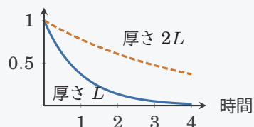
中心の温度 (1 項め)。2L は 4 倍 ゆっくり
