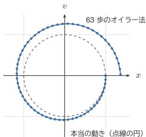
図1 ばねの状態の点 (x, v) 。目もりは \pm 1 で、点線の円は半径 1。本当は円を時計回りに 1 周してもとの点 (1, 0) にもどる (6-14)。63 歩のオイラー法 (点) は、1 歩ごとに少し外れずれ、うずをまいて (1.37, 0.03) に着く。
