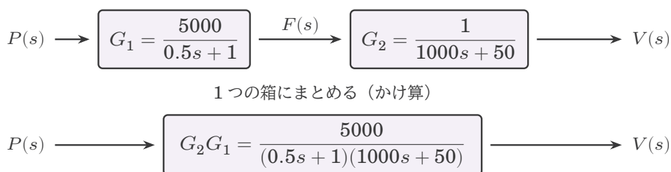
図 2 直列につないだ 2 つの箱は、伝達関数のかけ算の 1 つの箱になる。
