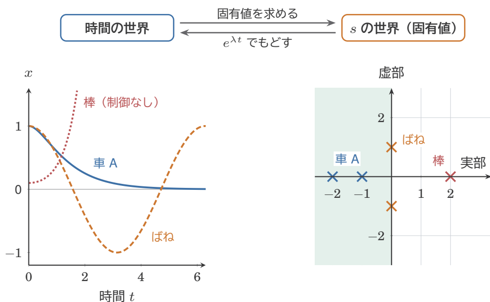
図3 左：車 A（実線、はじめ 1）、ばね（破線、はじめ 1）、手のひらの棒（点線、はじめ 0.1）の動き。右：それぞれの A の固有値（×）。うすい緑は実部が負の左半分。車 A の × は 2 つとも左半分で落ち着き、ばねはたての軸（虚軸）の上でゆれ続け、棒は +2 が右半分にあったおられる（棒のもう 1 つの固有値 -2 は、車 A の -2 と同じ場所）。
