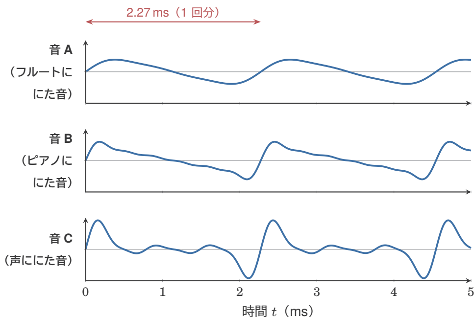
図1 同じ「ラ」（440 Hz）の3つの音の波形。横は時間（1 ms は1000分の1秒）、たては空気の圧力の変化で、3つとも同じ目もり。どれも2.27 msごとに同じ形をくり返すが、くり返す形がちがう（形がわかりやすいように作った例）。
