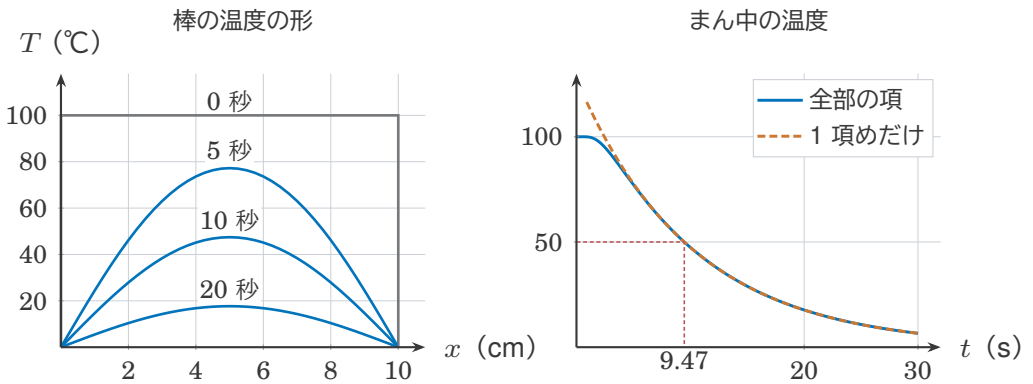
図 10 左：0・5・10・20 秒の形。時間とともに、角がとれて \sin の山の形 ( n = 1 の形) になり、そのまま小さくなる。右：まん中の温度。1 項めだけの線は、はじめは 100°C をこえる ( t = 0 で 127°C) が、すぐに全部の項の線と重なる。
