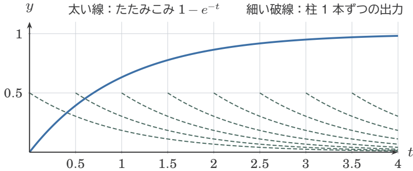
図7 入力 u = 1 （スイッチを入れたまま）を幅 0.5 の柱に分け、1 本ずつの出力 0.5e^{-(t-t_1)} （細い破線）を作る。柱を細くして、全部たした先が、太い線 1 - e^{-t} 。
