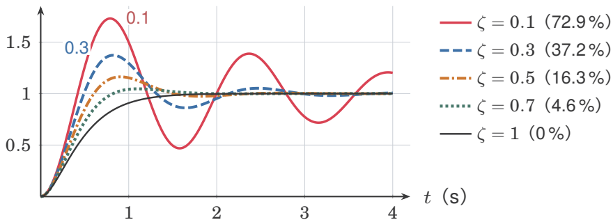
図8 2次おくれのステップの答え（ \omega_n = 4 \text{ rad/s} ）。右の見本の線の形と色で区別する（かっこの中は行きすぎ）。 \zeta が小さいほど、大きく行きすぎて、長くゆれる。
