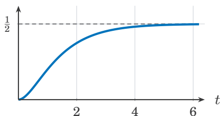
(1) \frac{1}{2} - e^{-t} + \frac{1}{2}e^{-2t}
