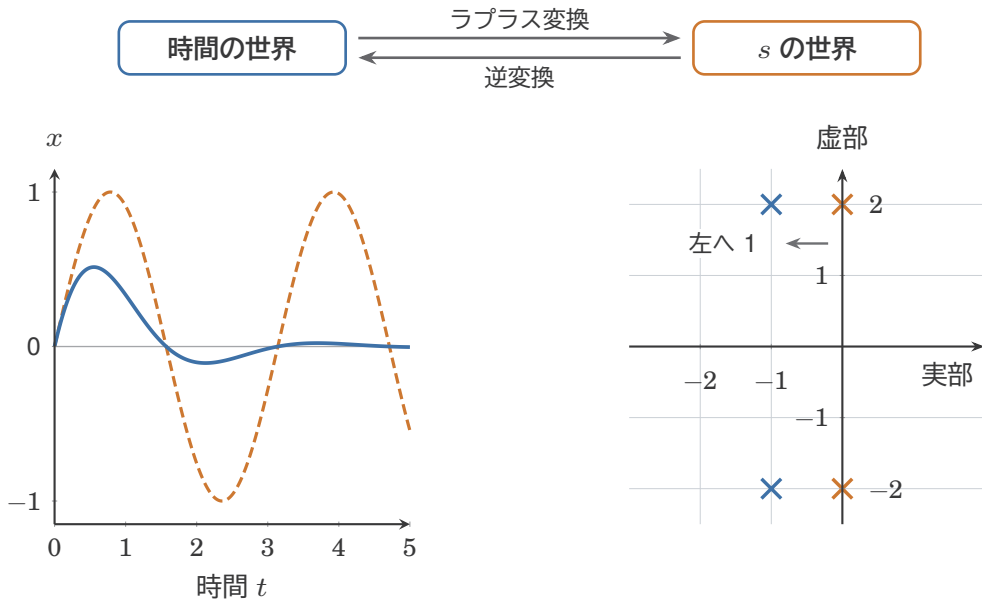
図2 左: \sin 2t (オレンジの破線) と e^{-t} \sin 2t (青い線)。右: それぞれの変換の分母が 0 になる所 (オレンジの×が \sin 2t 、青の×が e^{-t} \sin 2t )。 e^{-t} をかけると、×が左へ 1 だけずれる。
